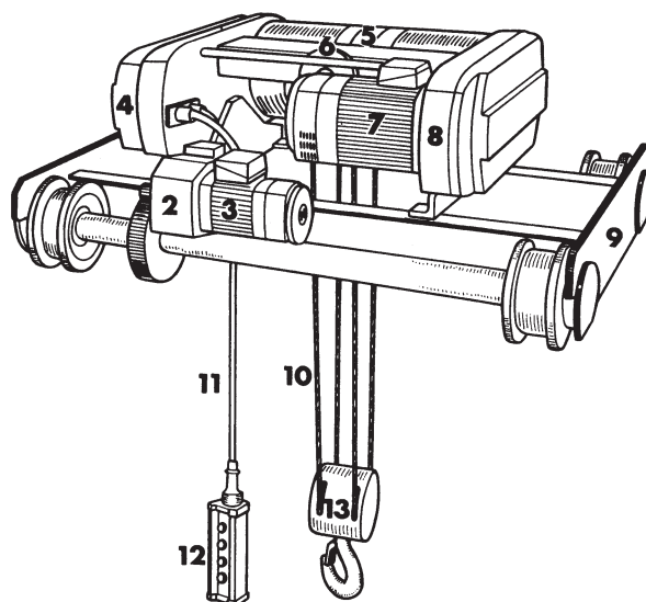
Telfertralla Hoist crab
