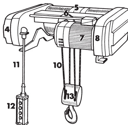
TMF TMF-F
